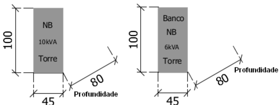
Figura05: Medidas Nobreak 10kVA torre;
