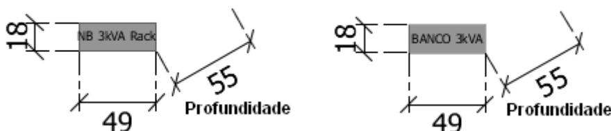
Figura02: Medidas Nobreak 3kVA Rack;
