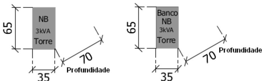
Figura01: Medidas Nobreak 3kVA Torre;
