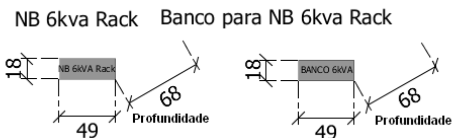
Figura04: Medidas Nobreak 6kVA Rack;
