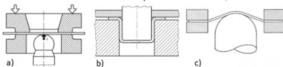
Figura 2: ensaios de embutimento. a) Erichsen e Olsen. b) Swift e c) Fukui
