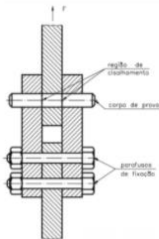
Figura 2: dispositivos de ensaio de cisalhamento, utilizando lâmina móvel e sistema de estampo
