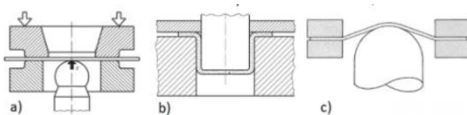
Figura 2: ensaios de embutimento. a) Erichsen e Olsen. b) Swift e c) Fukui
