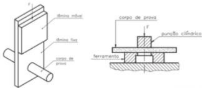
Figura 2: dispositivos de ensaio de cisalhamento, utilizando lâmina móvel e sistema de estampo
