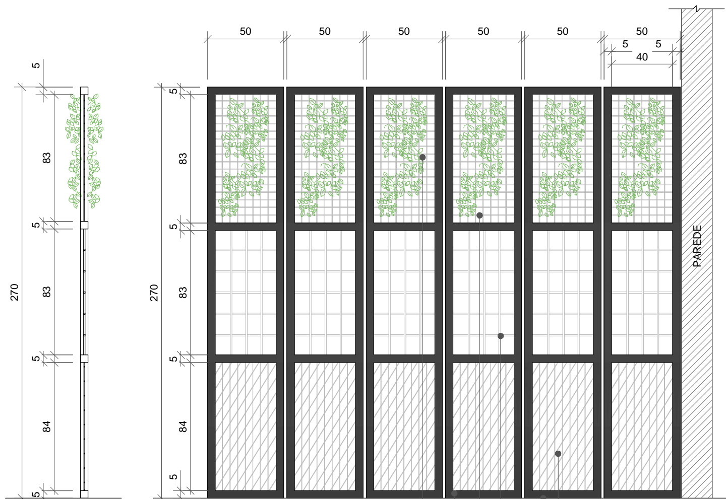
CORTE LATERAL ESC: 1/25
