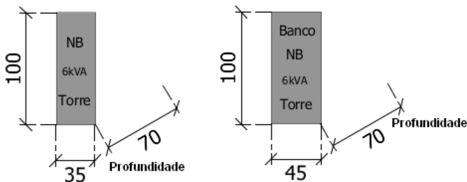
Figura03: Medidas Nobreak 6kVA Torre;
