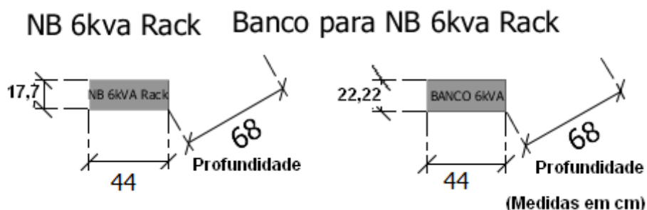
Figura04: Medidas Nobreak 6kVA Rack;
