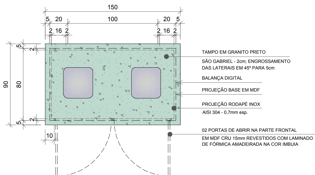
PLANTA BAIXA
