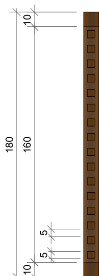
VISTA LATERAL
