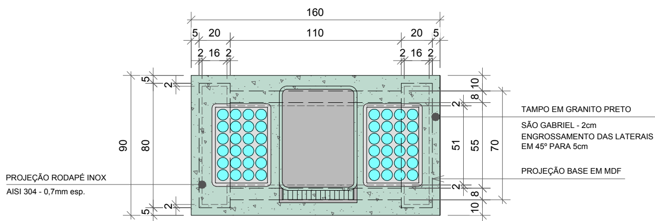
PLANTA BAIXA BALCÃO APOIO 02 - REFRESQUEIRA e COPOS
