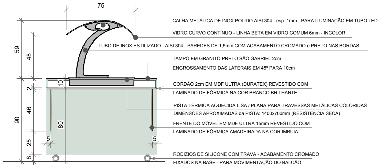
CORTE LATERAL
