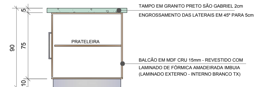
CORTE LATERAL
