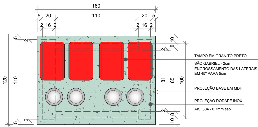
BALCÃO APOIO 01 PRATOS e BANDEJAS LINHA NORMAL
