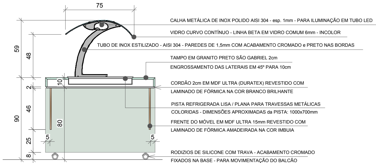
CORTE LATERAL
