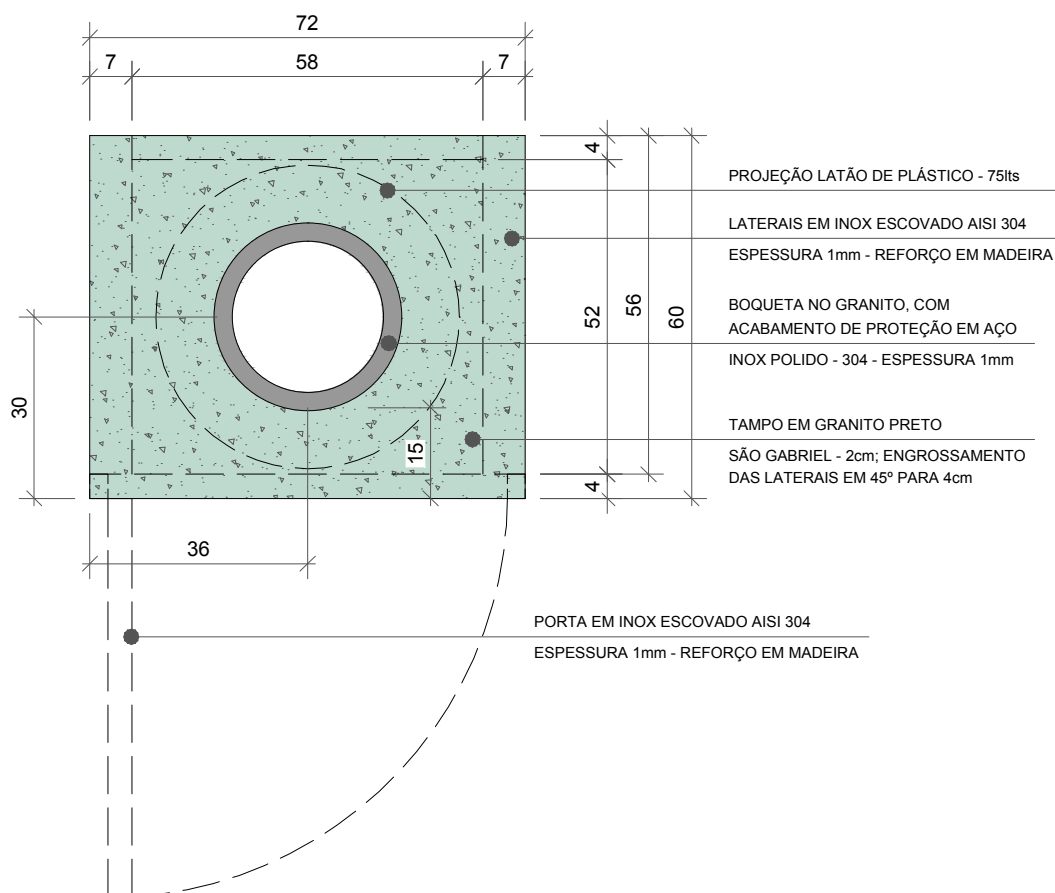
PLANTA BAIXA BALCÃO LIXOS / DETRITOS (02 unidades)
