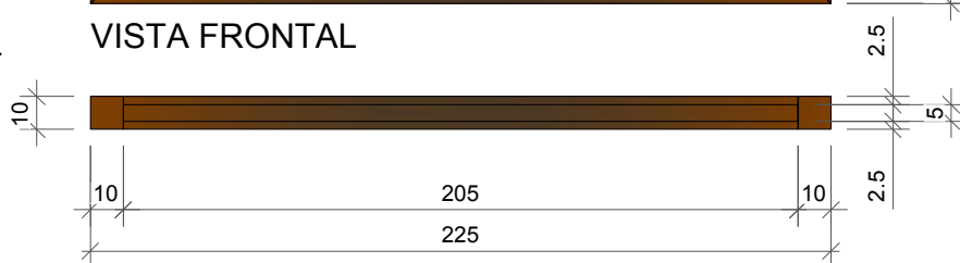
PLANTA BAIXA - PAINEL 02 (1 UNIDADE)
