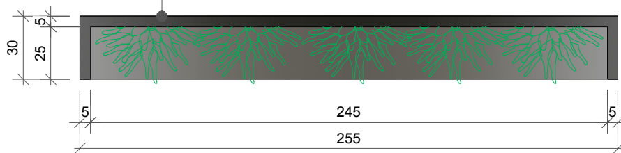
PLANTA BAIXA - PAINEL JARDIM VERTICAL 01 (01 UNIDADE)
