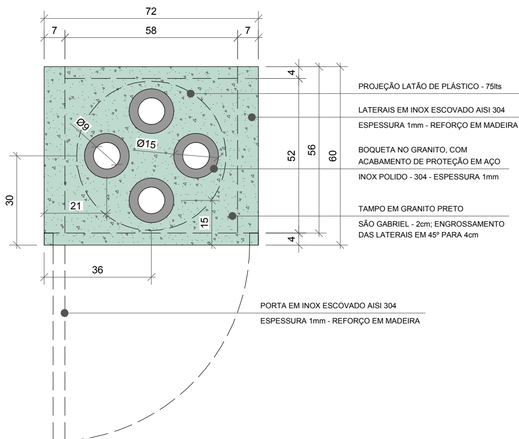
PLANTA BAIXA BALCÃO DESCARTÁVEIS (02 unidades)
